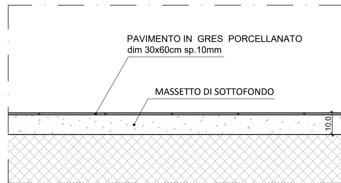
2 PAVIMENTO IN GRES PORCELLANATO SCALA 1:10
