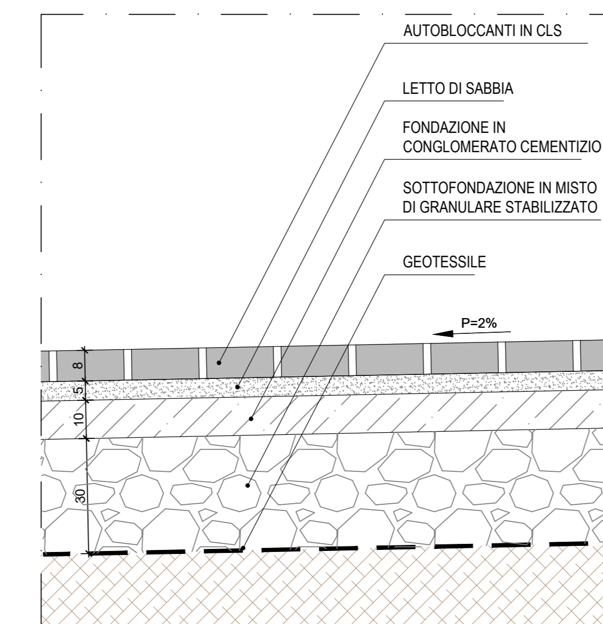
12 PAVIMENTAZIONE PERCORSO PEDONALE SCALA 1:10
