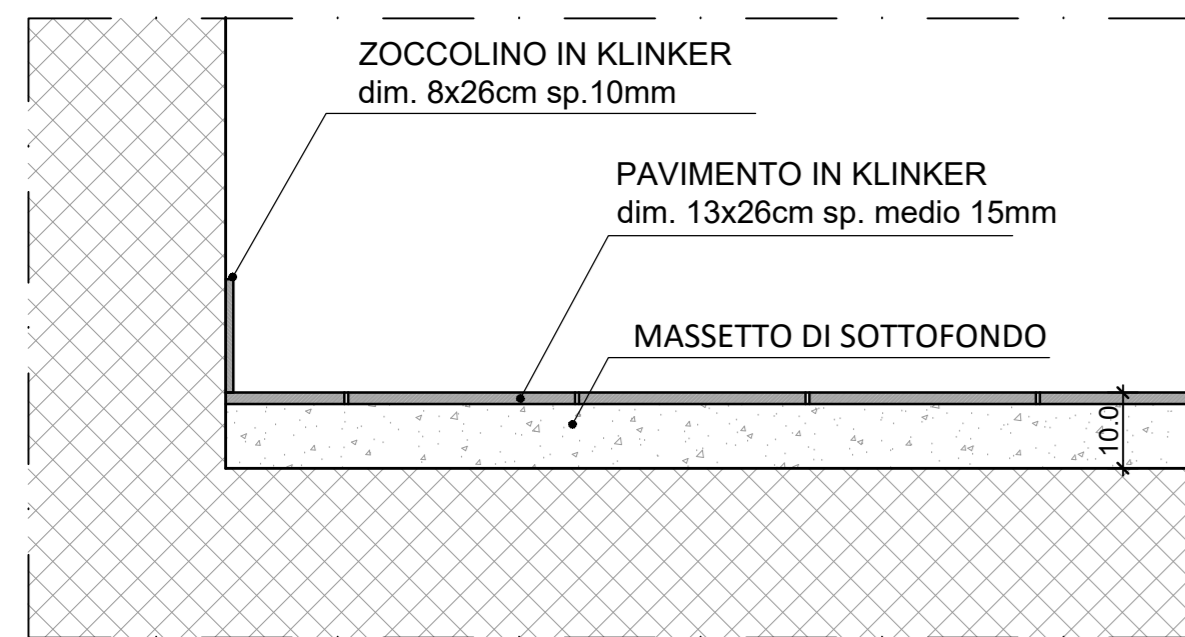
4 PAVIMENTO IN KLINKER SCALA 1:10
