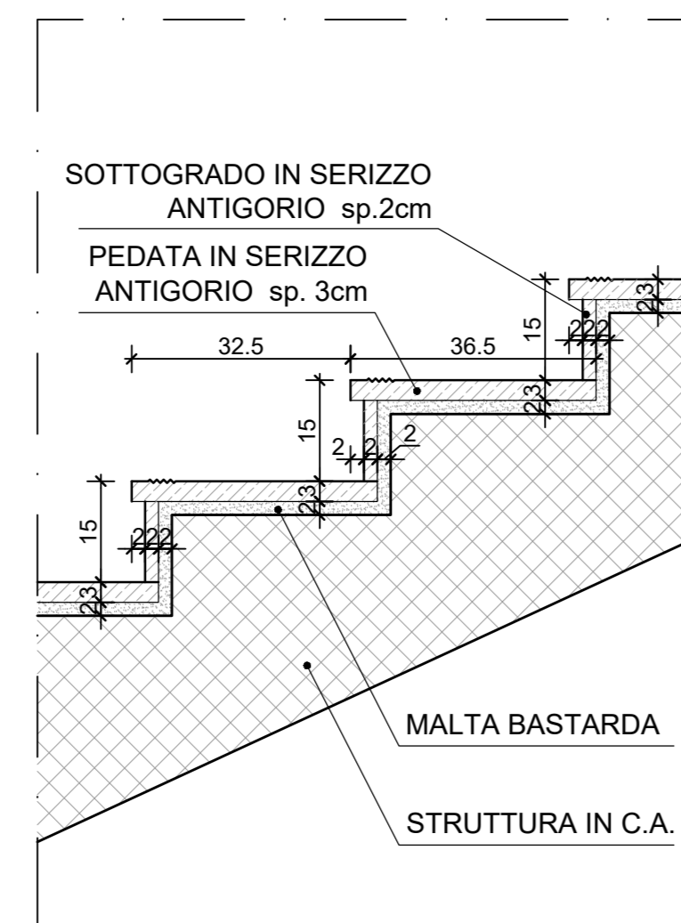
8 DETTAGLIO GRADINI IN SERIZZO ANTIGORIO SCALA 1:10
