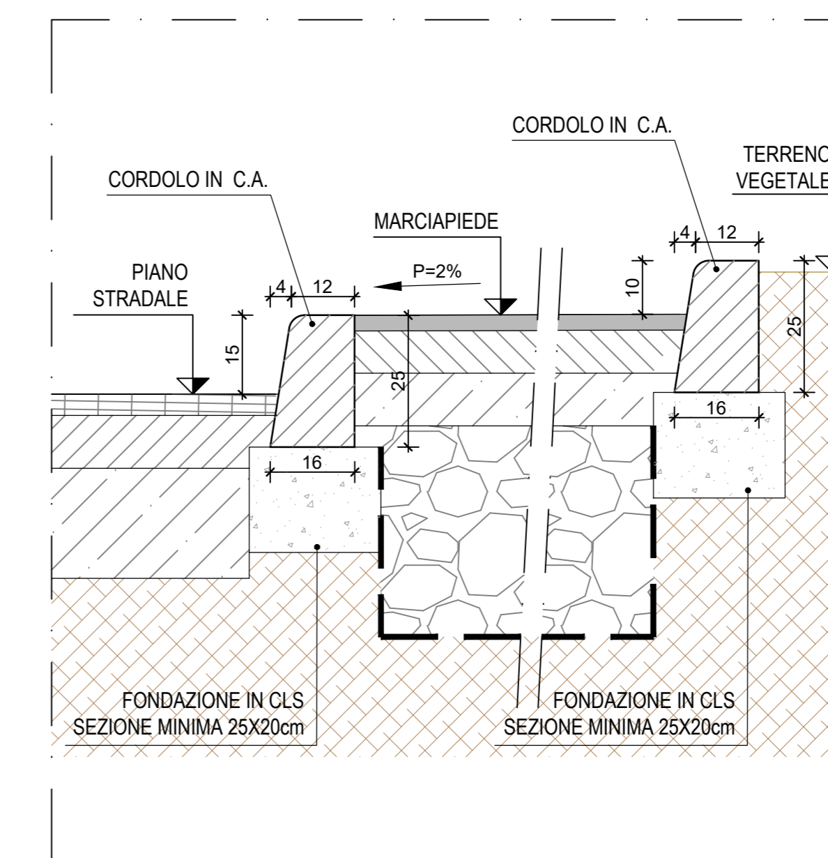
14 CORDOLI IN C.A. SU MARCIAPIEDI SCALA 1:10
