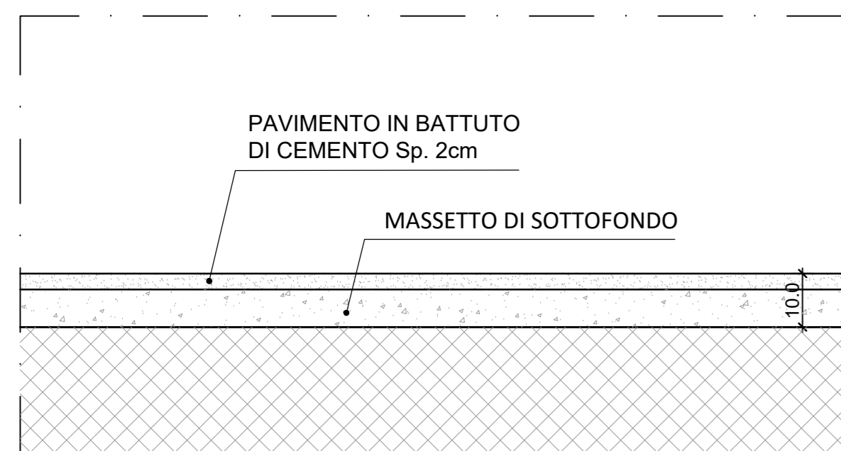
5 PAVIMENTO IN BATTUTO DI CEMENTO SCALA 1:10
