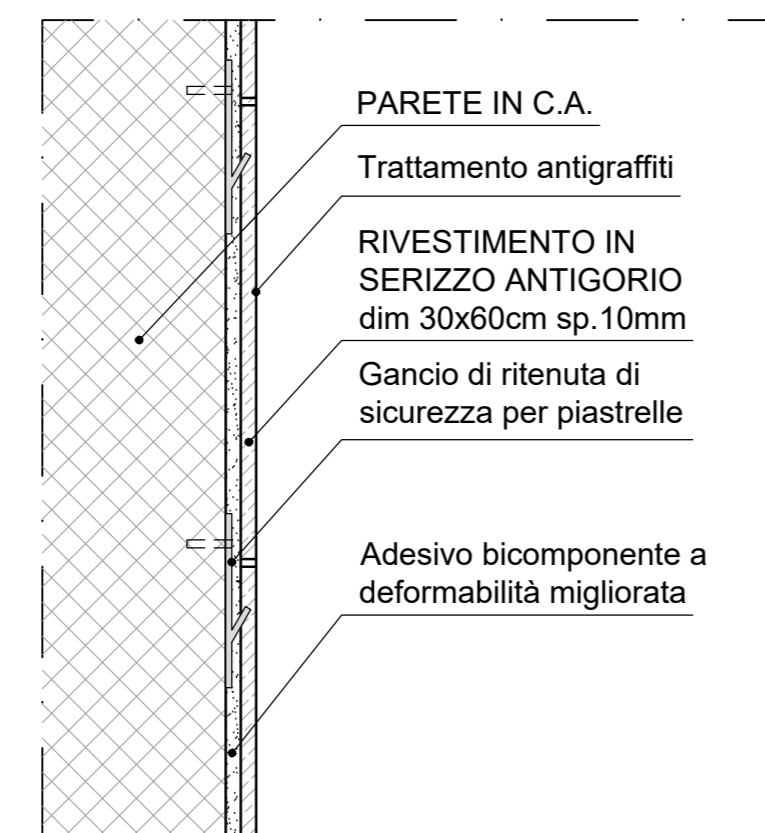
7 PARETE RIVESTITA IN SERIZZO ANTIGORIO SCALA 1:5
