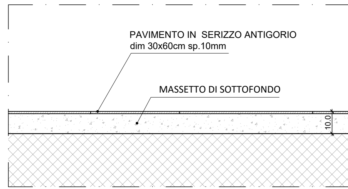
1 PAVIMENTO IN SERIZZO ANTIGORIO SCALA 1:10
