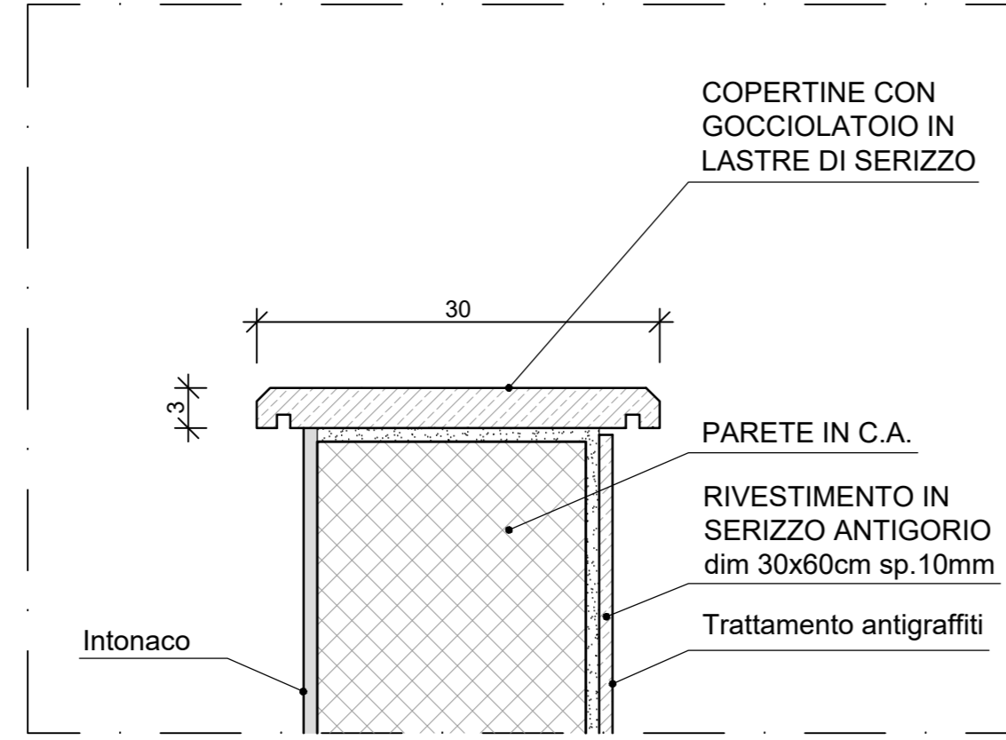
6 DETTAGLIO COPERTINE ACCESSI FERMATE SCALA 1:5
