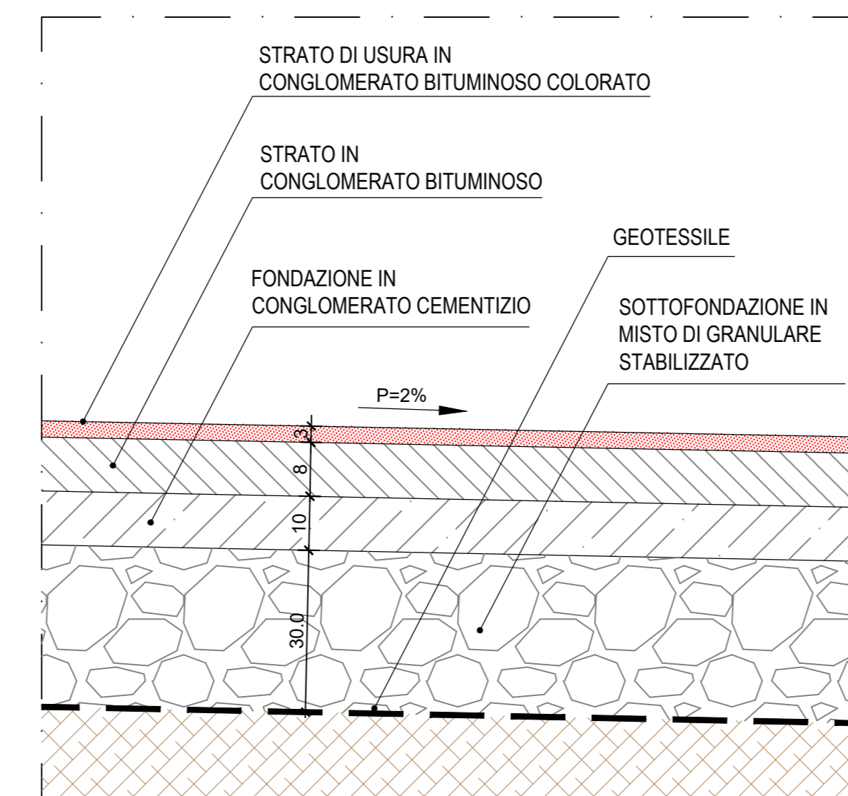
12 PAVIMENTAZIONE PERCORSO PEDONALE SCALA 1:10
