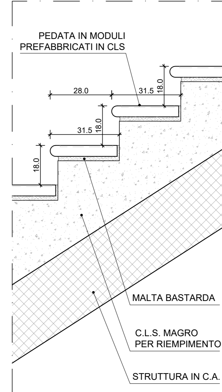
9 GRADINI CON MODULI PREFABBRICATI IN CLS SCALA 1:10
