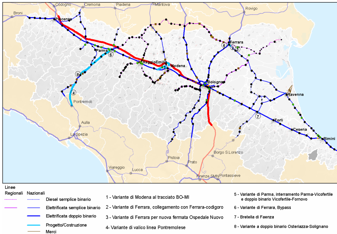
Figura. Schema rete ferroviaria di previsione al 2020
