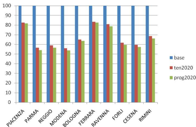
Figura. Valore relativo della concentrazione media annuale di NO 2 nei comuni capoluogo dell'Emilia-Romagna, fatto 100 il valore attuale.
