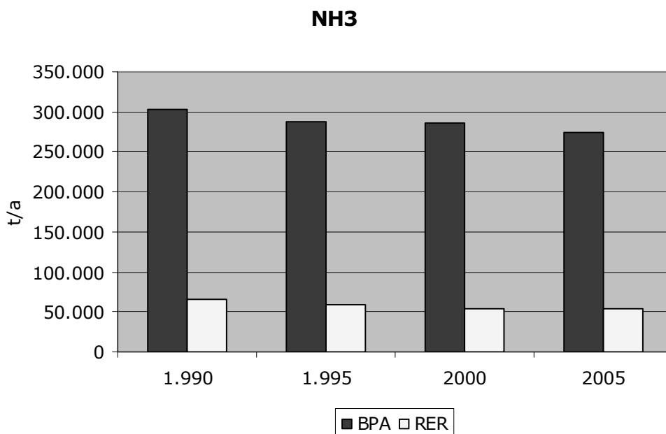
Figura. Trend emissioni BPA-RER di NH3 – dati APAT-ISPRA
