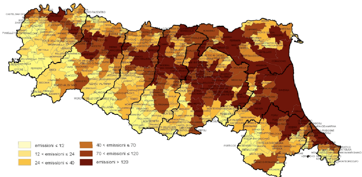
Figura Scenario programmatico 2020, emissioni di NOx complessive da traffico per comune
