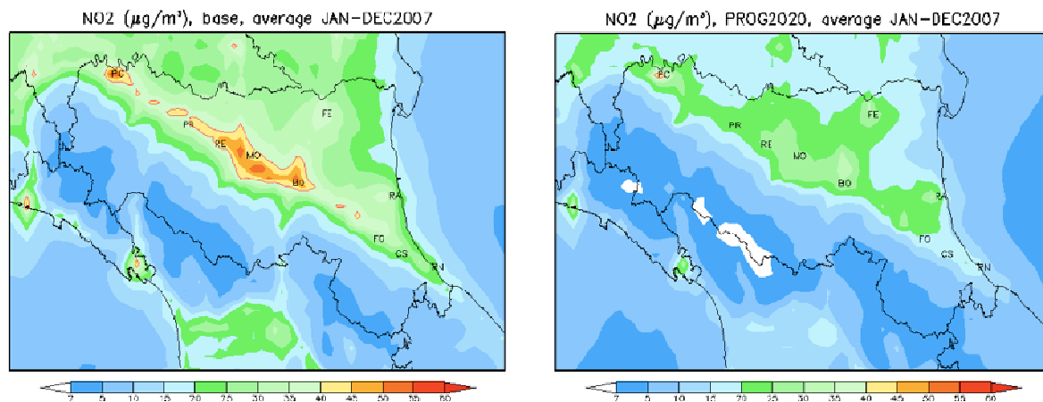
Figura. Concentrazione media annuale di biossido di azoto ( \text{NO}_2 ) in Emilia-Romagna. A sinistra lo scenario di riferimento, a destra lo scenario programmatico 2020. La linea rossa evidenzia le aree all'interno delle quali viene superato il valore limite di 40 \mu\text{g}/\text{m}^3 in vigore dal 2010.
