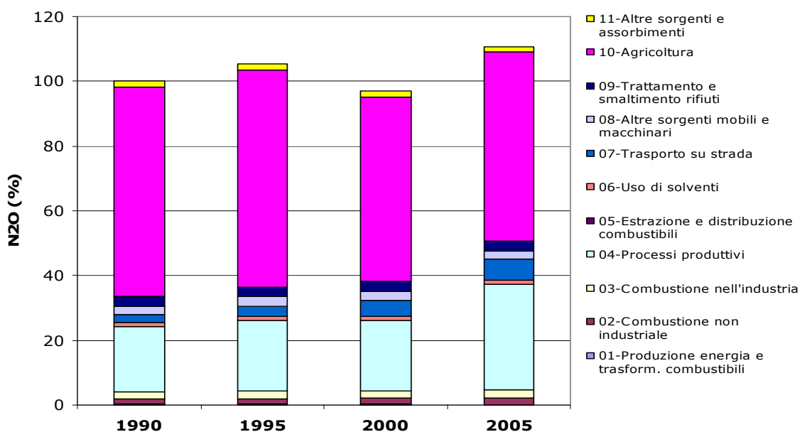
Figura - Emissioni % rispetto al 1990 di N2O (Mt/a) per macrosettore CORINAIR – Regione Emilia-Romagna Fonte APAT-ISPRA
