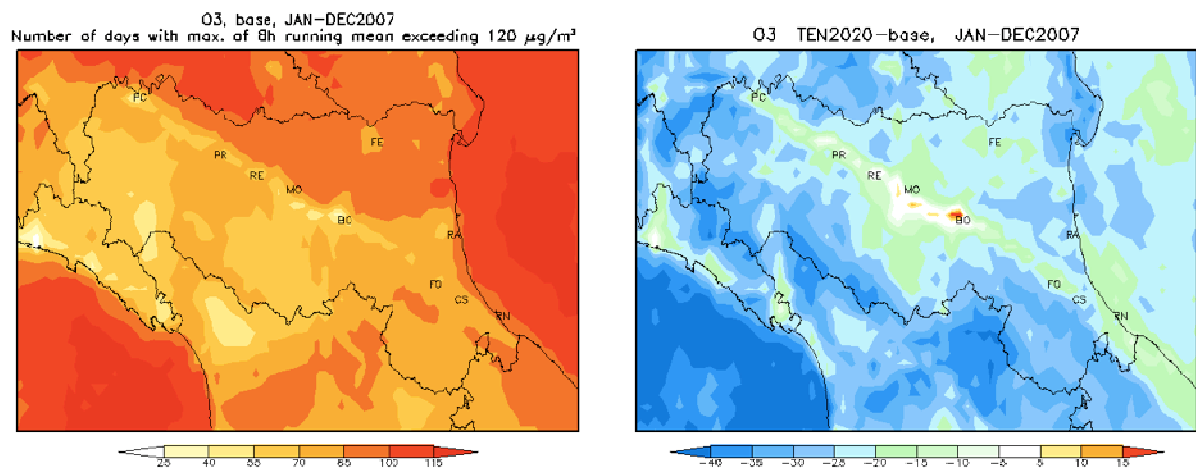
Figura. Numero di giorni in cui il massimo della media mobile di ozono (O 3 ) in Emilia-Romagna supera i 120 µg/m 3 . Il valore bersaglio per la protezione della salute è 25 superamenti l'anno. A sinistra lo scenario di riferimento, a destra le differenze dello scenario tendenziale al 2020 rispetto allo scenario di riferimento.
