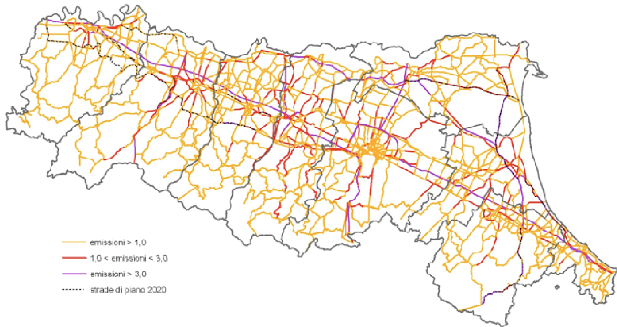
Figura. Scenario programmatico, emissioni di PM10 lineari, cioè dovute agli spostamenti assegnati a ciascun arco stradale, gli archi previsti al 2020 sono indicati in tratteggio.
