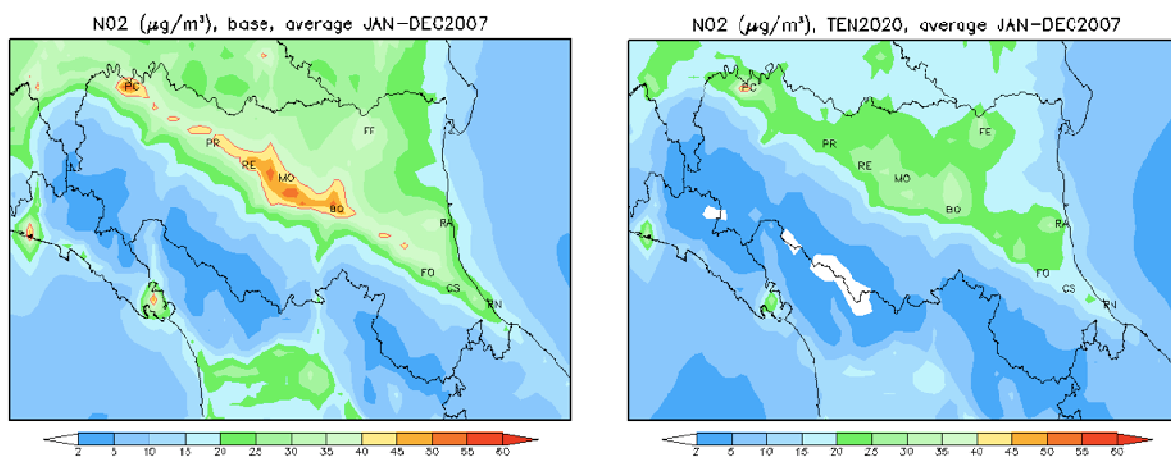
Figura. Scenario di riferimento 2007 (sinistra) e scenario tendenziale 2020 (destra). Concentrazione media annuale di biossido di azoto (NO 2 ) in Emilia-Romagna. La linea rossa evidenzia le aree all'interno delle quali viene superato il valore limite di 40 \mu\text{g}/\text{m}^3 in vigore dal 2010.
