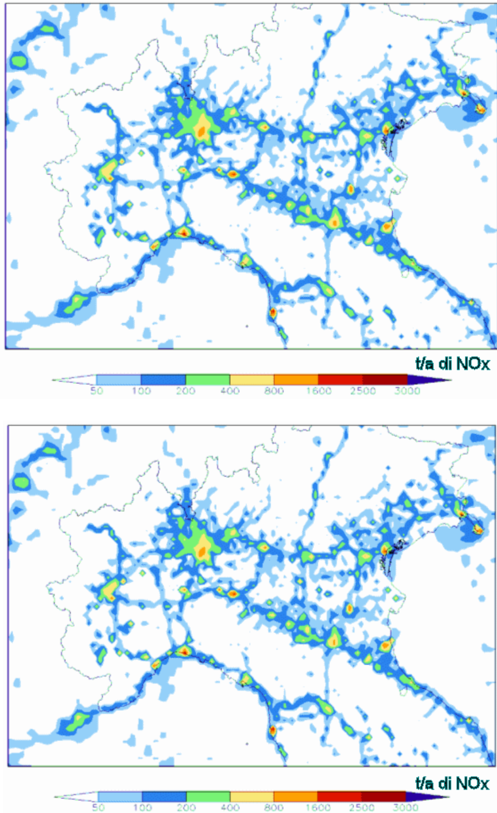
Figura. Emissioni annuali di NOx relative agli scenari emissivi 2020 tendenziale (in alto) e programmatico (in basso).
