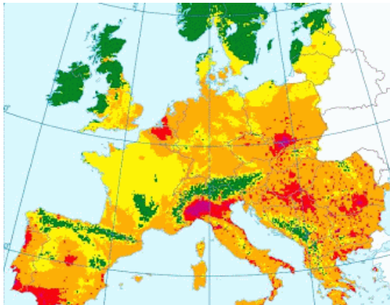
Figura. inquinamento da polveri sottili in Europa. Le regioni più inquinate sono evidenziate in rosso: emerge con chiarezza la criticità della Pianura Padana [Agenzia europea per l'Ambiente, 2006]
