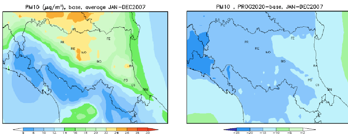
Figura. Concentrazione media annuale di PM10 in Emilia-Romagna. A sinistra scenario di riferimento, a destra variazioni percentuali scenario programmatico al 2020.
