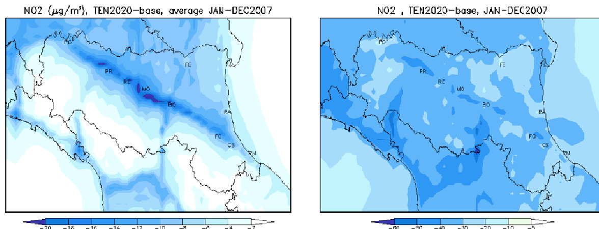
Figura. Differenze di concentrazione media annuale di biossido di azoto (NO 2 ) in Emilia-Romagna tra lo scenario tendenziale e quello di riferimento. A sinistra il valore assoluto, a destra in percentuale.
