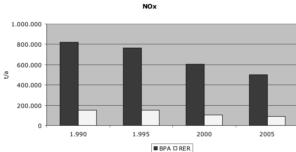
Figura. Trend emissioni BPA-RER di NOx – dati APAT-ISPRA
