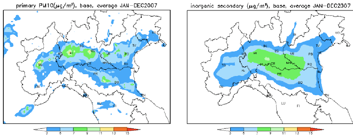
Figura. Scenario di riferimento 2007. Concentrazioni medie annuali della frazione primaria (a sinistra) e della frazione inorganica secondaria (a destra) di PM10 [ \mu\text{g}/\text{m}^3 ].
