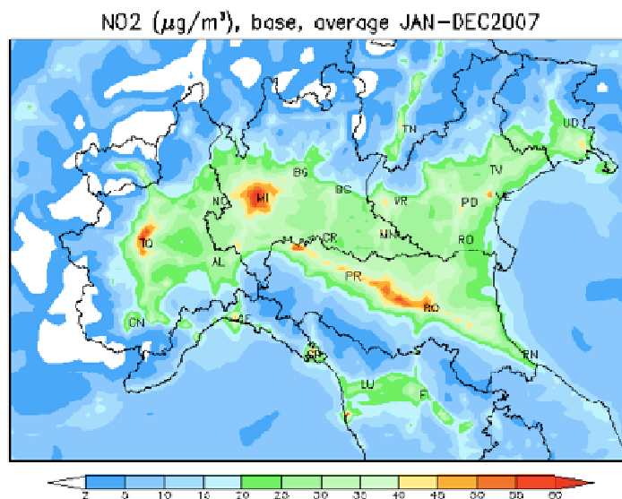
Figura. Scenario di riferimento 2007. Concentrazioni medie annuali di NO 2 .
