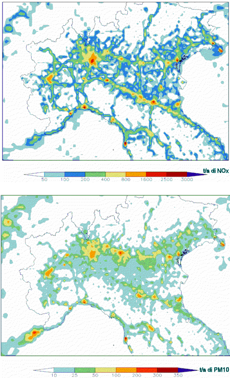
Figura. Emissioni annuali di NOx (in alto) e di PM10 (in basso) nello scenario di riferimento (t/anno)
