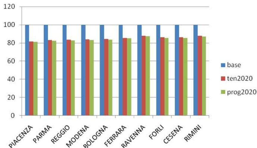
Figura. Valore relativo della concentrazione media annuale di PM10 nei comuni capoluogo dell'Emilia-Romagna, fatto 100 il valore attuale
