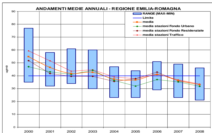
Figura. Medie annuali del PM10 in Emilia-Roimagna
