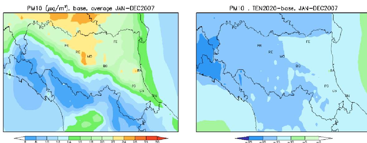
Figura. Concentrazione media annuale di PM10 in Emilia-Romagna. A sinistra lo scenario di riferimento, a destra variazioni percentuali dello scenario tendenziale al 2020 rispetto a quello di riferimento.
