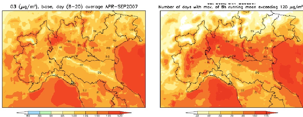
Figura. Scenario di riferimento 2007. Concentrazioni di ozono. A sinistra le medie diurne estive (fascia oraria 8-20); a destra il numero di giorni in cui il massimo della media mobile supera i 120 µg/m 3 .
