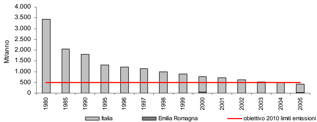
Figura - Emissioni di ossidi di zolfo (SOx) (Annuario dati ambientali; dati ISPRA)
