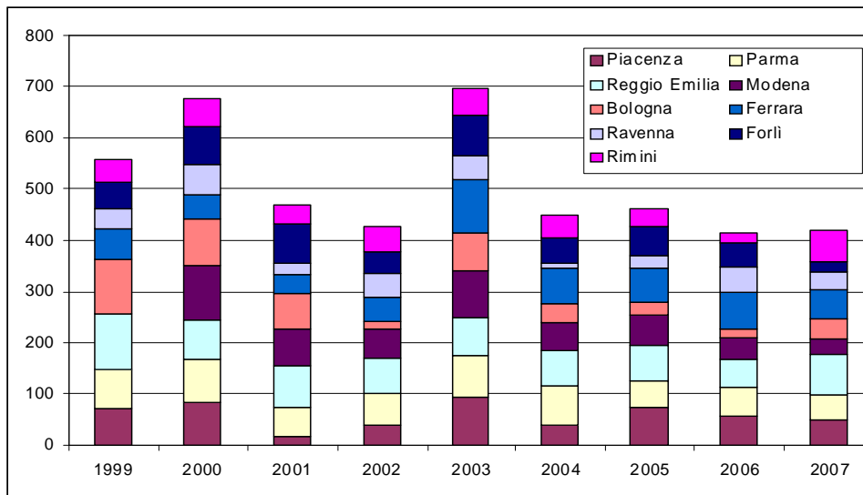
Figura. Ozono (O3) in Emilia-Romagna: giorni di superamento dell'obiettivo a lungo termine per la salute umana (120 µg/m3).(Arpa Emilia-Romagna. 2008)
