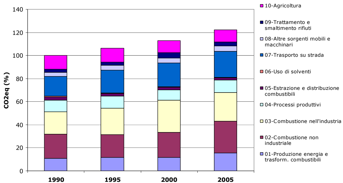
Figura - Emissioni % rispetto al 1990 di CO 2 eq (Mt/a) per macrosettore CORINAIR – Regione Emilia-Romagna, Fonte APAT-ISPRA
