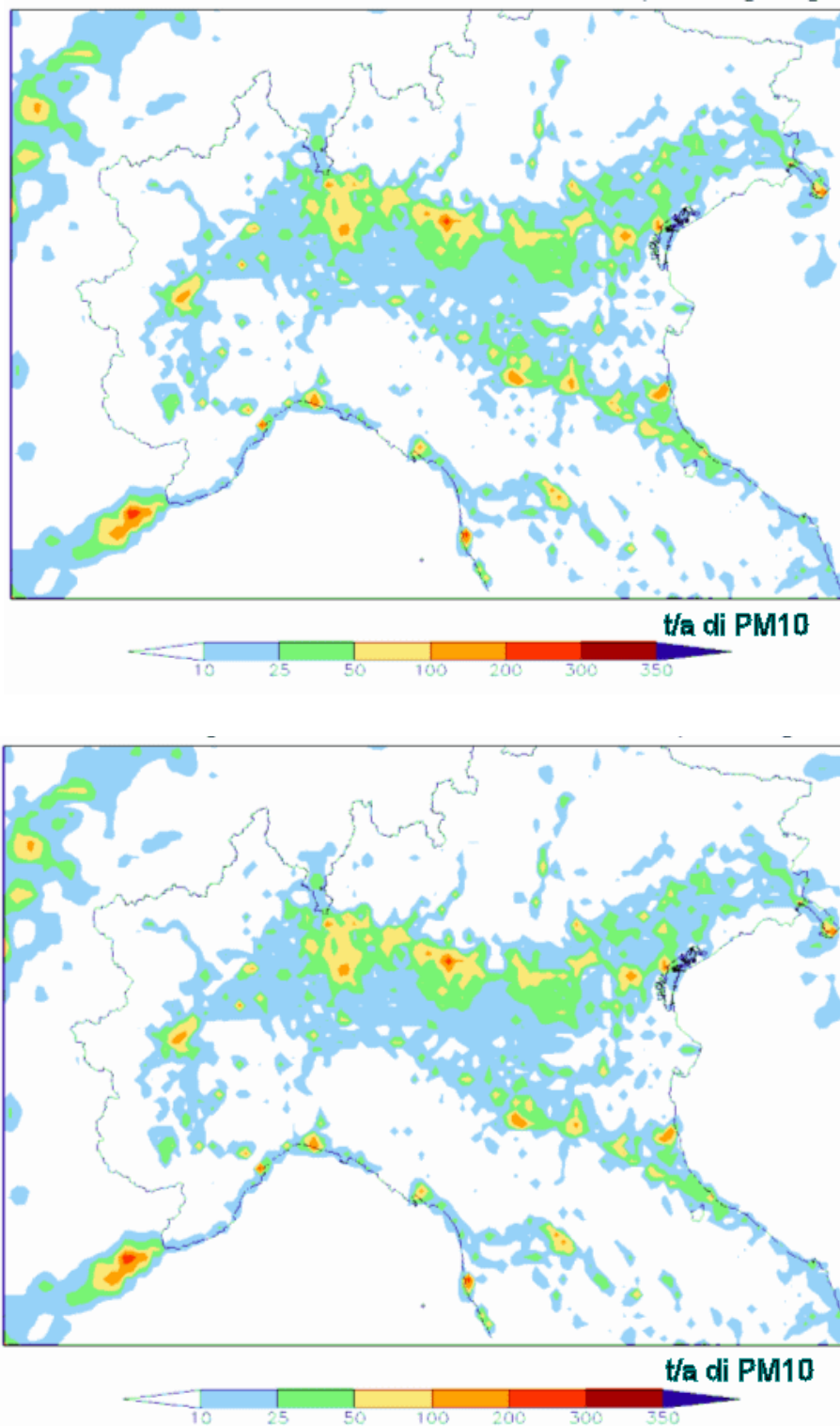
Figura. Emissioni annuali di PM10 relative agli scenari emissivi 2020 tendenziale (in alto) e programmatico (in basso).
