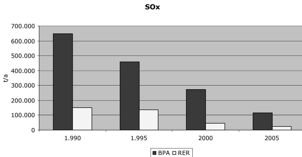
Figura. Trend emissioni BPA-RER di SOx – dati APAT-ISPRA
