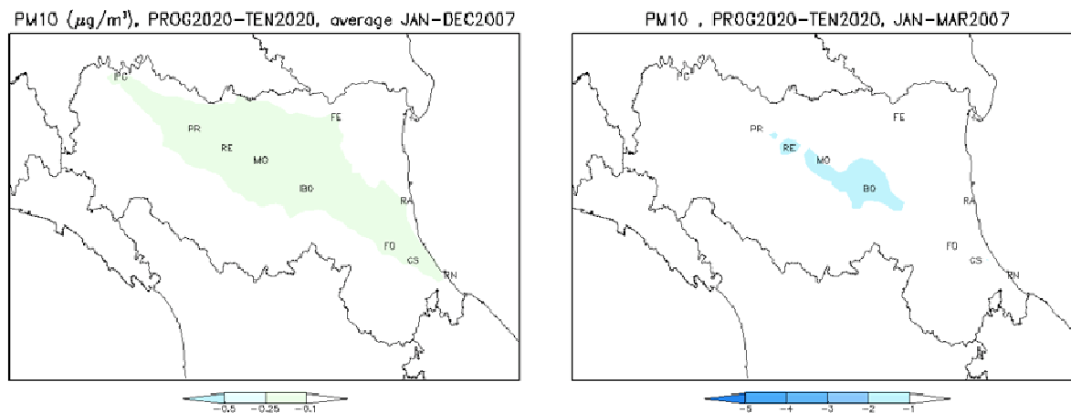
Figura. Differenze di concentrazione media di PM10 in Emilia-Romagna tra lo scenario programmatico al 2020 e quello tendenziale. A sinistra il valore assoluto, a destra in percentuale.
