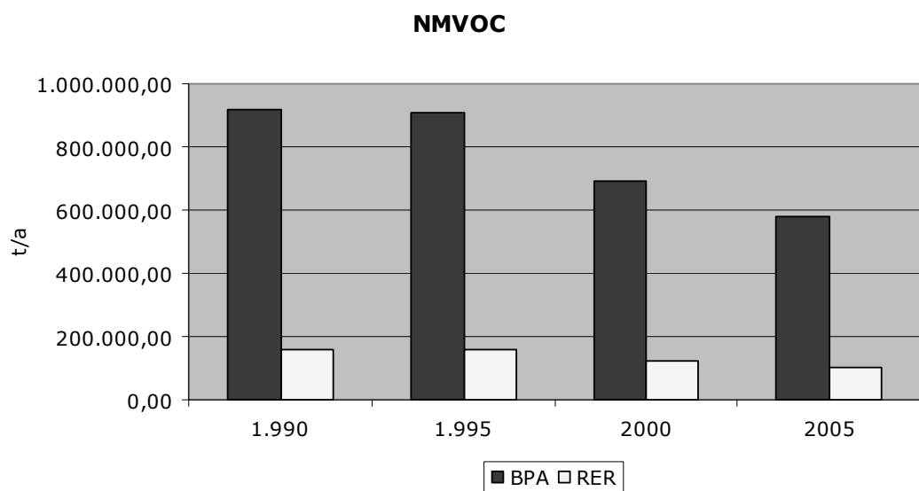
Figura. Trend emissioni BPA-RER di NMVOC – dati APAT-ISPRA
