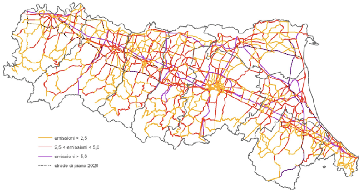
Figura. Scenario programmatico emissioni di NOx lineari, cioè dovute agli spostamenti assegnati a ciascun arco stradale, gli archi previsti al 2020 sono indicati in tratteggio.
