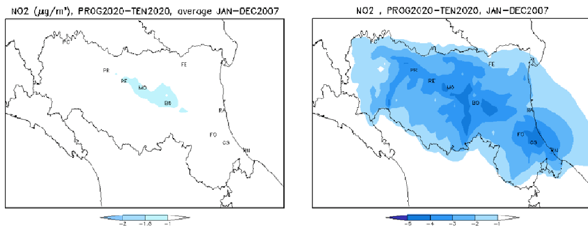
Figura. Differenze di concentrazione media di biossido di azoto ( \text{NO}_2 ) in Emilia-Romagna tra lo scenario programmatico al 2020 e quello tendenziale. A sinistra il valore assoluto, a destra in percentuale.
