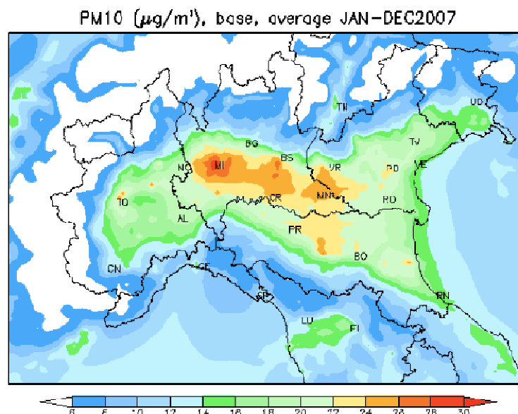
Figura. Scenario di riferimento 2007. Concentrazioni medie annuali di PM10 [ \mu\text{g}/\text{m}^3 ].
