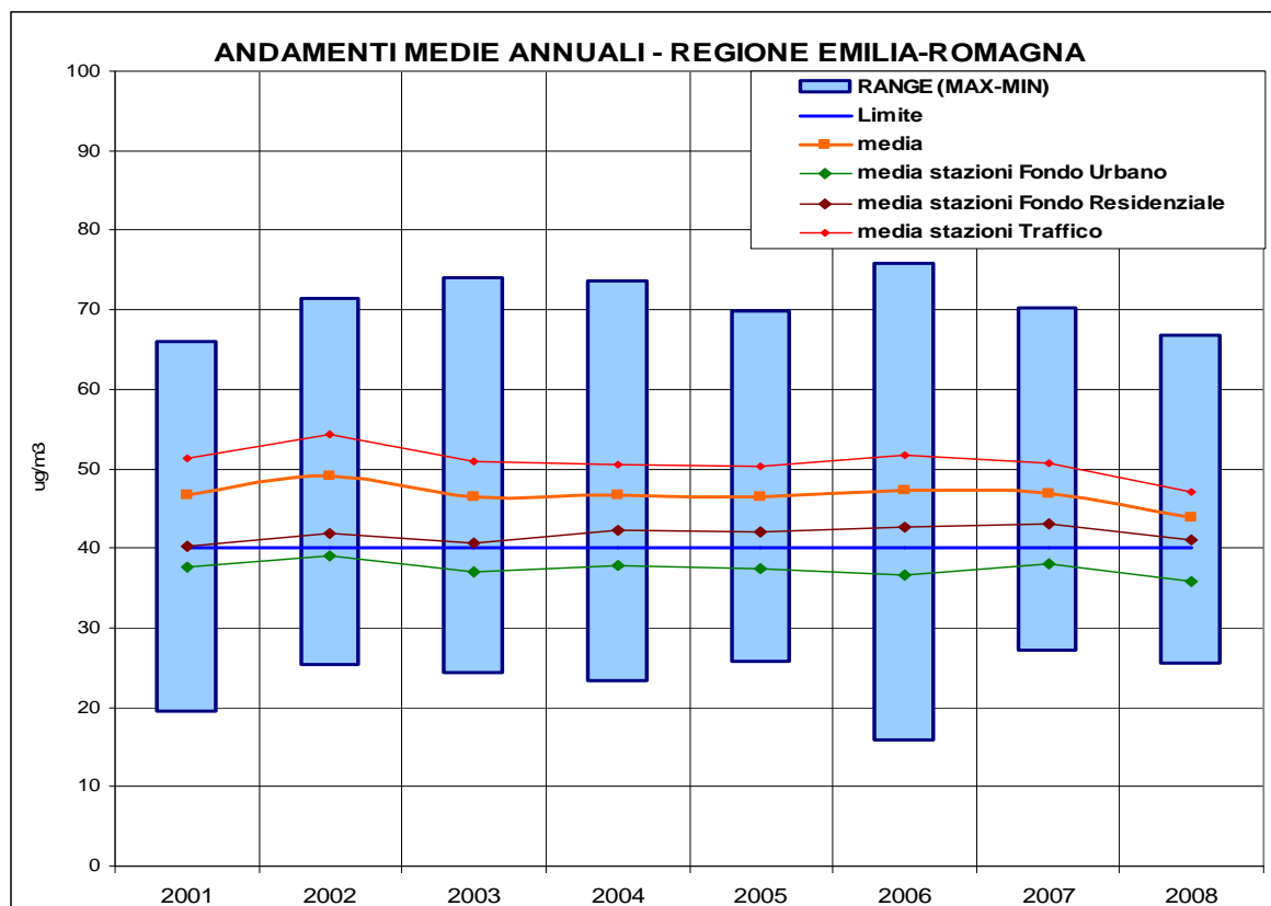
Figura. Medie annuali di NO2 in Emilia-Roimagna
