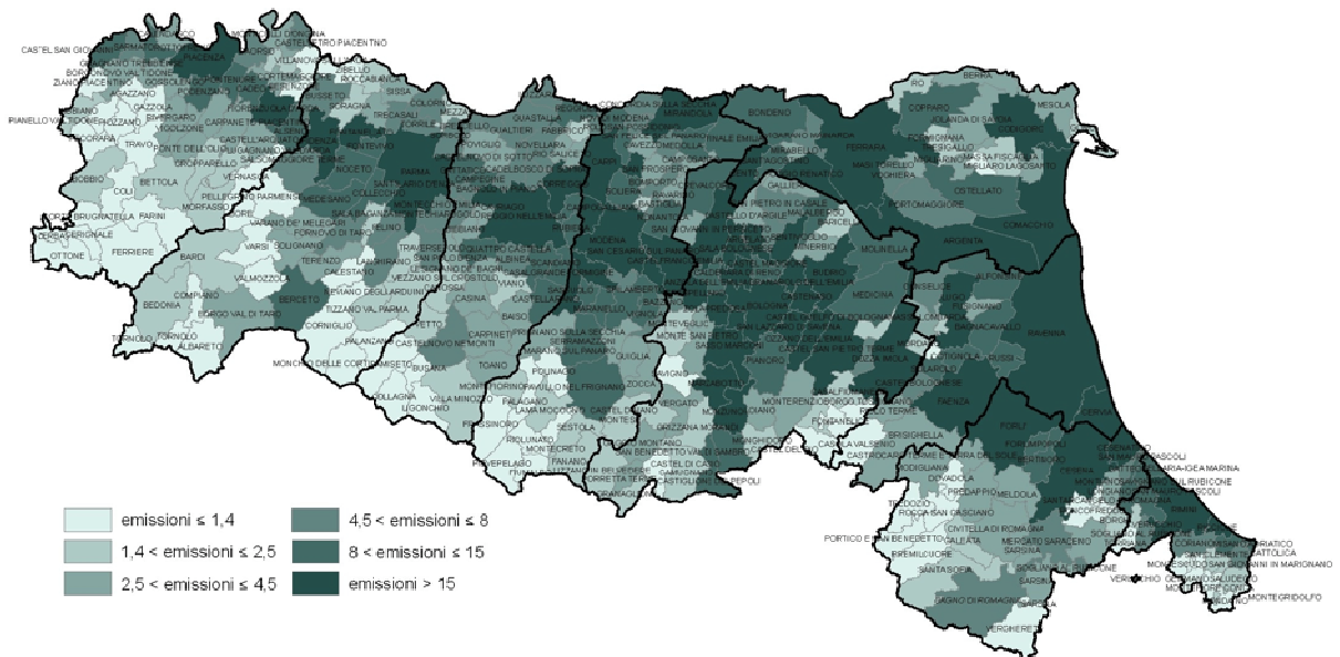
Figura. Scenario programmatico 2020, emissioni di PM10 complessive da traffico per comune
