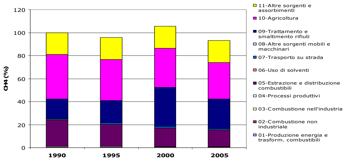
Figura - Emissioni % rispetto al 1990 di CH 4 (Mt/a) per macrosettore CORINAIR – Regione Emilia-Romagna Fonte APAT-ISPRA
