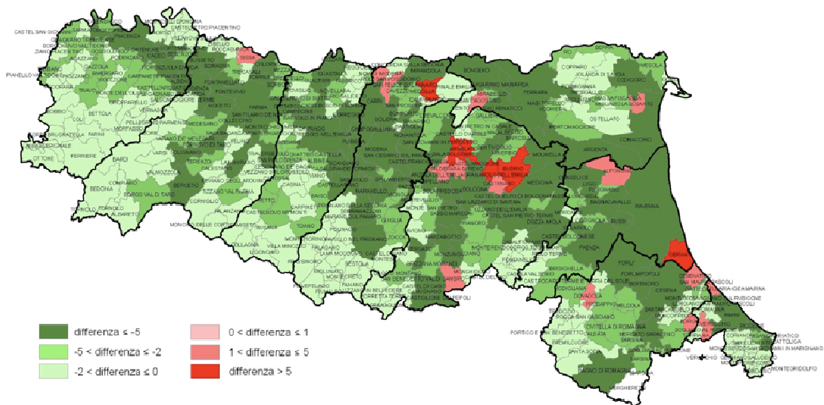
Figura. Differenza di emissioni di PM10 tra gli scenari di riferimento-2007 e programmatico-2020 (in verde sono indicate le riduzioni di emissione nello scenario programmatico-2020).
