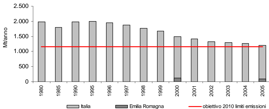
Figura - Emissioni composti organici volatili non metanici (NMVOC) (Annuario dati ambientali; dati ISPRA)
