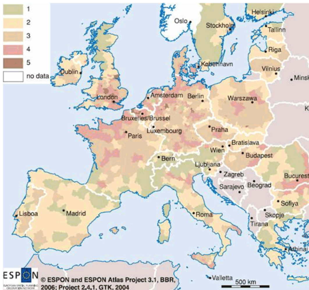
Figura. Livelli di frammentazione ecologica. I livelli di frammentazione delle aree naturali indicano proporzioni tra ambiti naturali frammentare ed ambiti naturali omogenei (ESPON, 2004)
