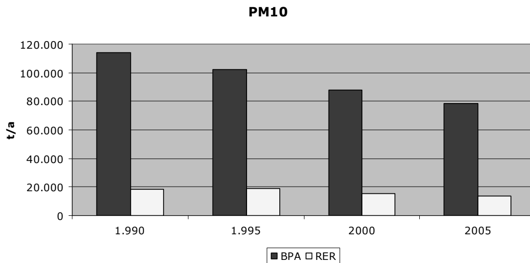
Figura. Trend emissioni BPA-RER di polveri sottili PM10– dati APAT-ISPRA
