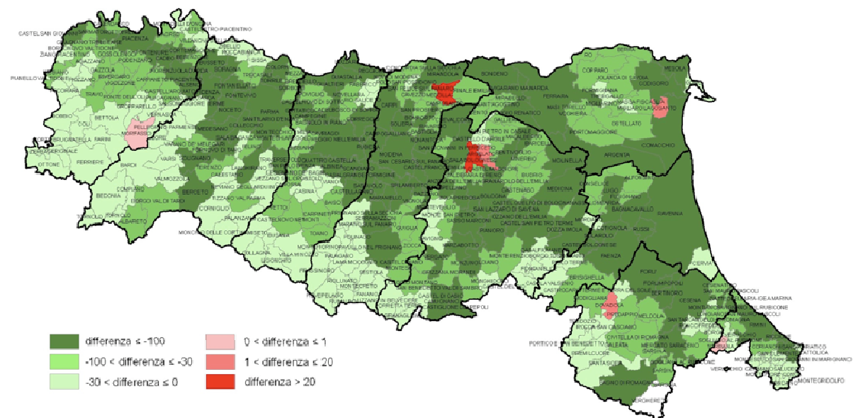
Figura. Differenza di emissioni di NOx tra gli scenari di riferimento-2007 e programmatico-2020 (in verde sono indicate le riduzioni di emissione nello scenario programmatico-2020).
