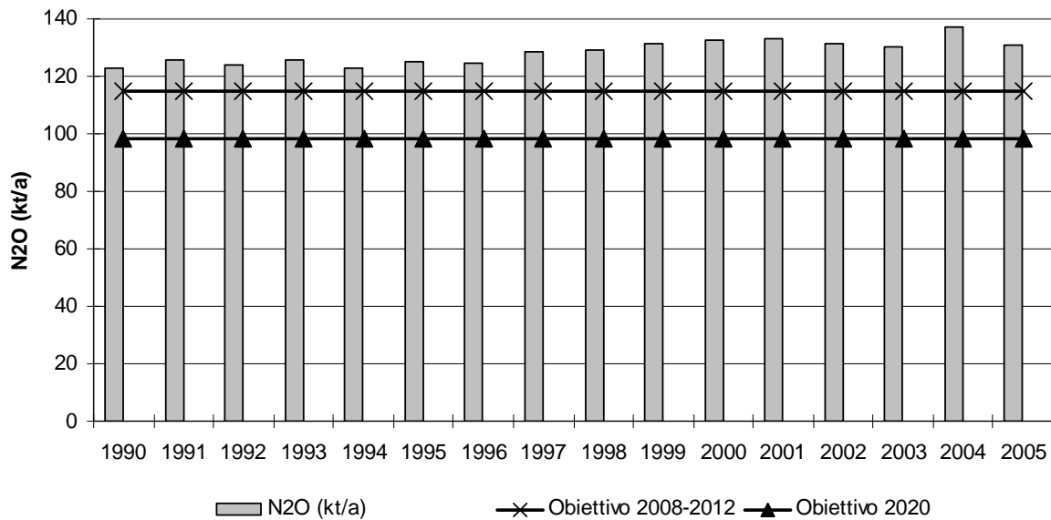
Figura - Trend delle emissioni nazionali di N2O (kt/a) – Fonte APAT-ISPRA
