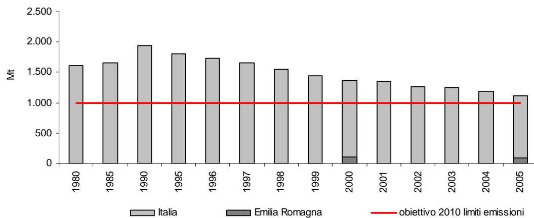
Figura - Emissioni di ossidi di azoto (NOx) (Annuario dati ambientali; dati ISPRA)
