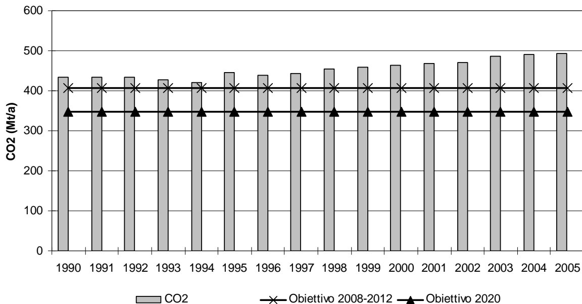
Figura - Trend delle emissioni nazionali di CO2 (Mt/a) – Fonte APAT-ISPRA
