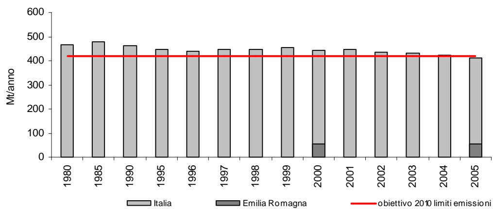
Figura. Emissioni di ammoniaca (NH3) (Annuario dati ambientali; dati ISPRA)
