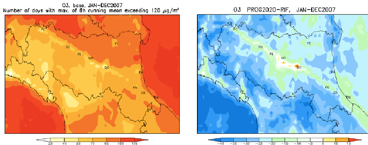
Figura. Numero di giorni in cui il massimo della media mobile di ozono ( O_3 ) in Emilia-Romagna supera i 120 \mu\text{g}/\text{m}^3 . Il valore bersaglio per la protezione della salute è 25 superamenti l'anno. A sinistra lo scenario di riferimento, a destra le differenze dello scenario programmatico al 2020 rispetto allo scenario di riferimento.
