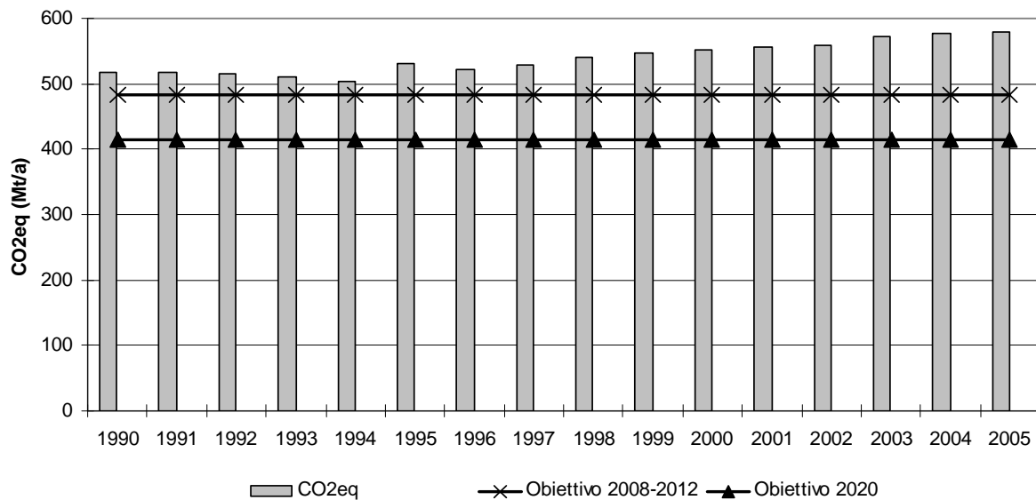
Figura - Trend delle emissioni nazionali di CO2 equivalente (Mt/a) – Fonte APAT-ISPRA
