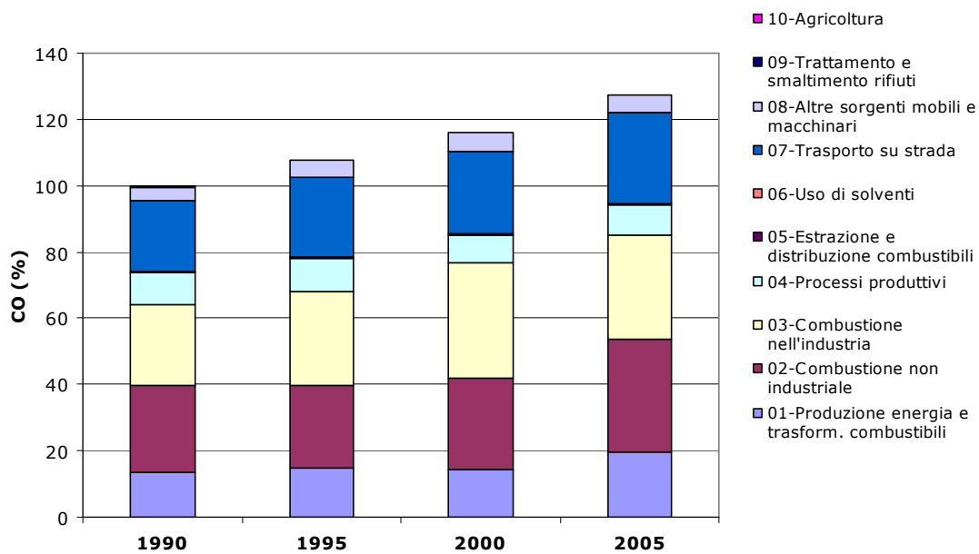
Figura - Emissioni % rispetto al 1990 di CO 2 (Mt/a) per macrosettore CORINAIR – Regione Emilia-Romagna Fonte APAT-ISPRA
