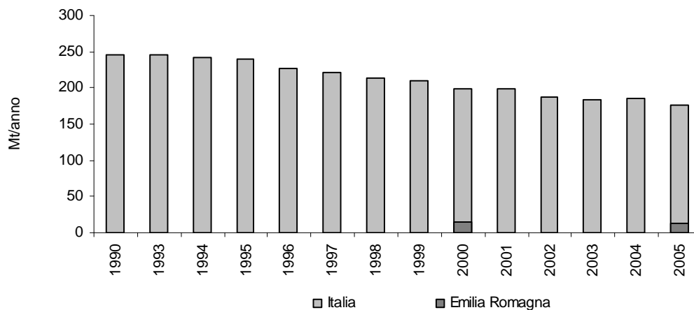
Figura. Emissioni di polveri sottili (PM10) (Annuario dati ambientali; dati ISPRA)
